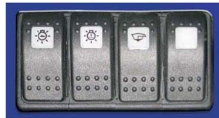
Приборная панель NorthSilver 605 слева направо: а) Вкл. ходового огня б) Вкл. якорного огня в) Вкл. водоотливной помпы г) Вкл. топливного индикатора и разъёма дополнительного электрооборудования
