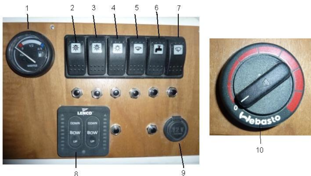
Приборная панель NorthSilver 690
