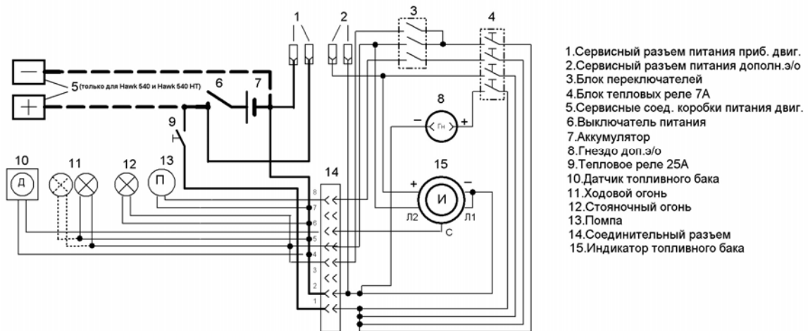
Схема подключения гнезда доп. э/о
